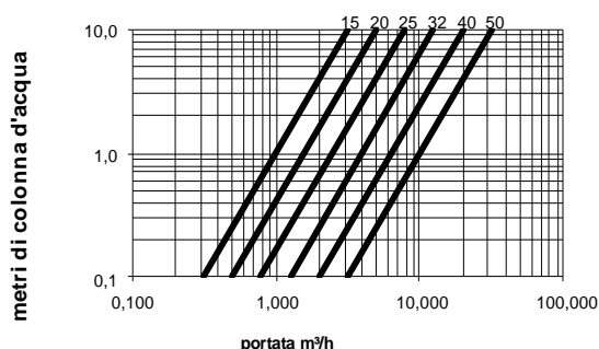
Diagramma delle perdite di carico
